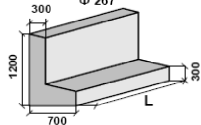
Фундаментные блоки Ф5, Ф6, Ф7
