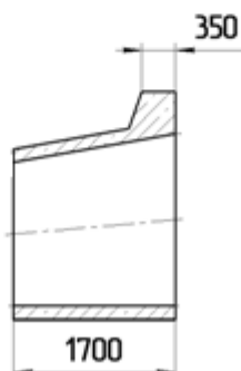
Коническое звено
