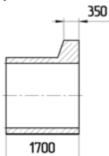
Звено с плоским опирание / Звено средней части
