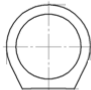
Звено с плоским опирание / Звено средней части
